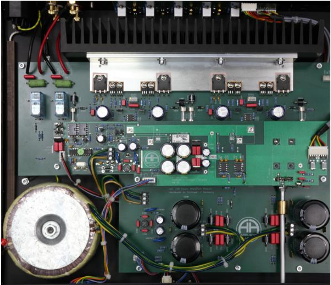
Power ES 的前級放大電路與後級功率輸出完全分離，分置不同的電路板上。狹長的上層是前級，下層則是後級，一方面妥善利用空間，另一方面則可減少干擾。
